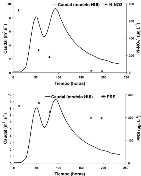
Figura 11. Hidrograma y concentración de nitrato y PRS correspondientes al evento de precipitación-caudal de marzo de 2001 en el arroyo Durazno (tomado de Arreghini et al. , -2-).
